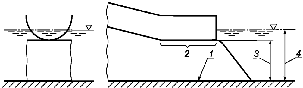
1 — дно бассейна; 2 — финишная секция/участок трассы спуска; 3 — расстояние от нижнего конца финишной секции/участка до дна бассейна; 4 — глубина воды
