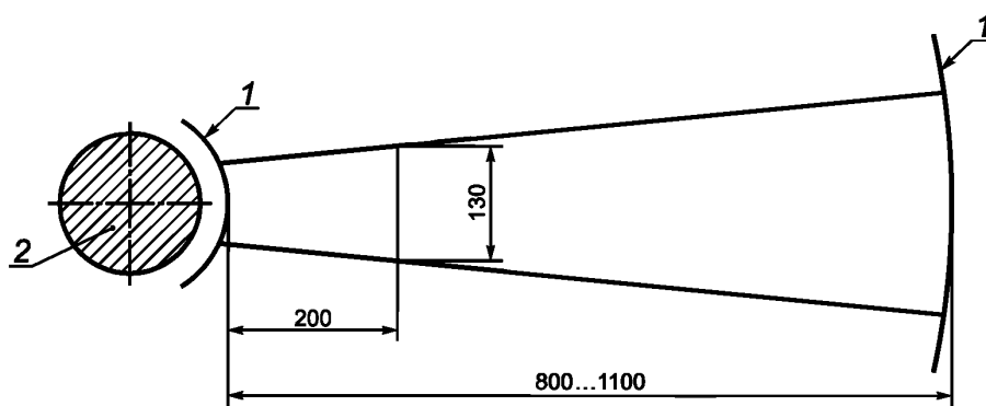
Рисунок 5 — Размеры винтовых или спиральных лестниц
