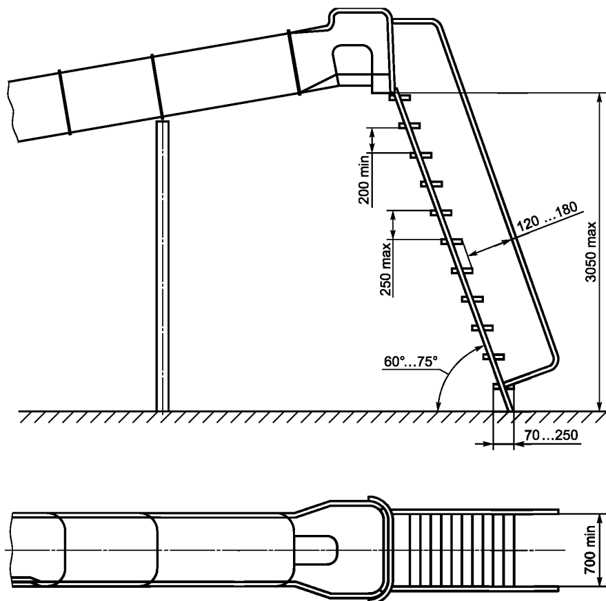
Рисунок 4 — Лестница-стремянка для подъема на водную горку
