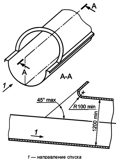
Рисунок 9 — Перекрытие начальной секции трассы спуска
