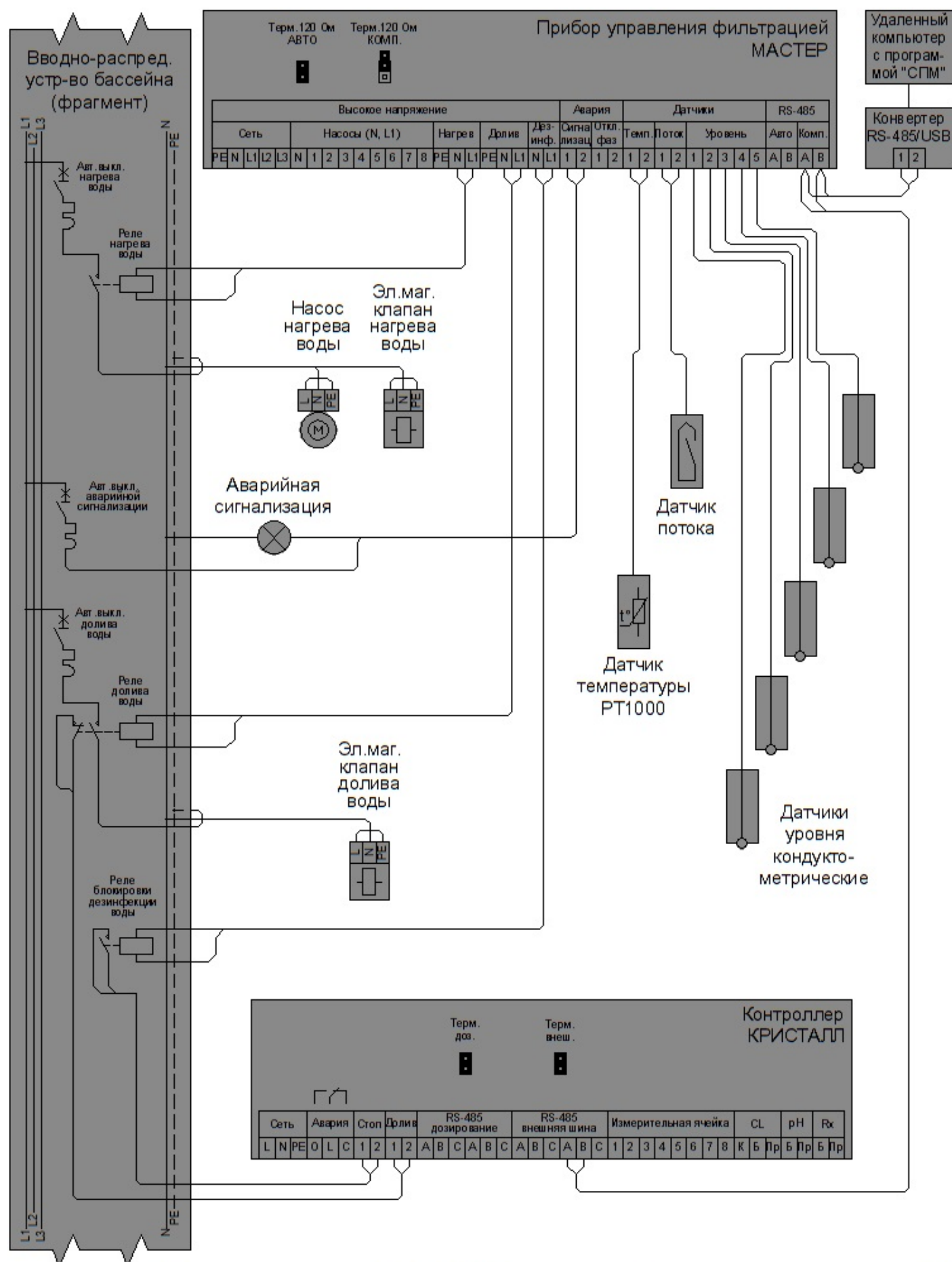
Схема подключения к прибору МАСТЕР нагрева, дезинфекции, долива, сигнализации и ПК
