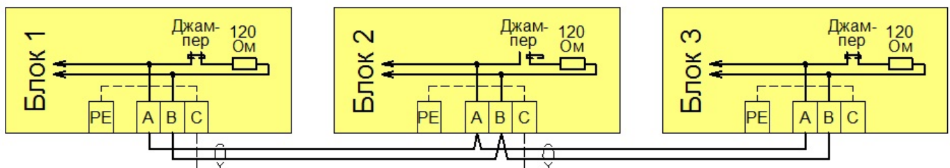
Рис.4.3-2 Соединение блоков для создания шины обмена данными RS-485
