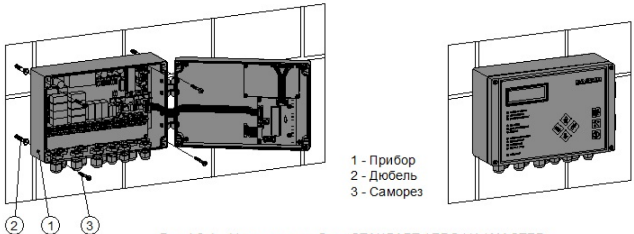
Рис. 4.2-1 Установка прибора СТАНДАРТ / ПРОФИ / МАСТЕР
