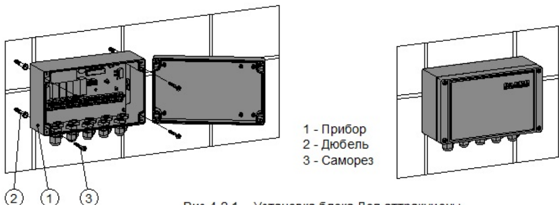
Рис.4.2-1 Установка блока Доп.аттракционы
